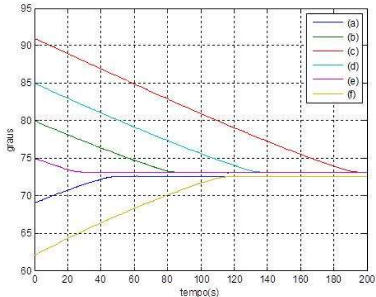
Figura 3: Gráfico da posição angular inicial com diferentes simulações: (a)= 69°; (b)=80°; (c)=91°, (d)=85°, (e)=75° e (f)=62°.
