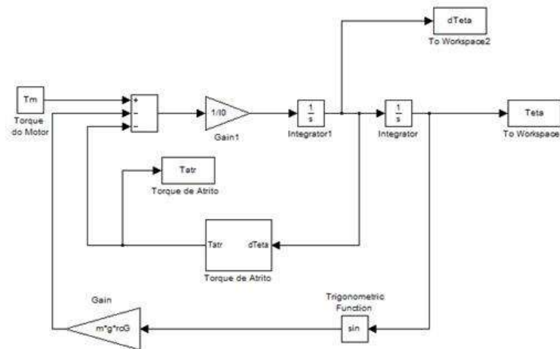
Figura 2: Diagrama de blocos
